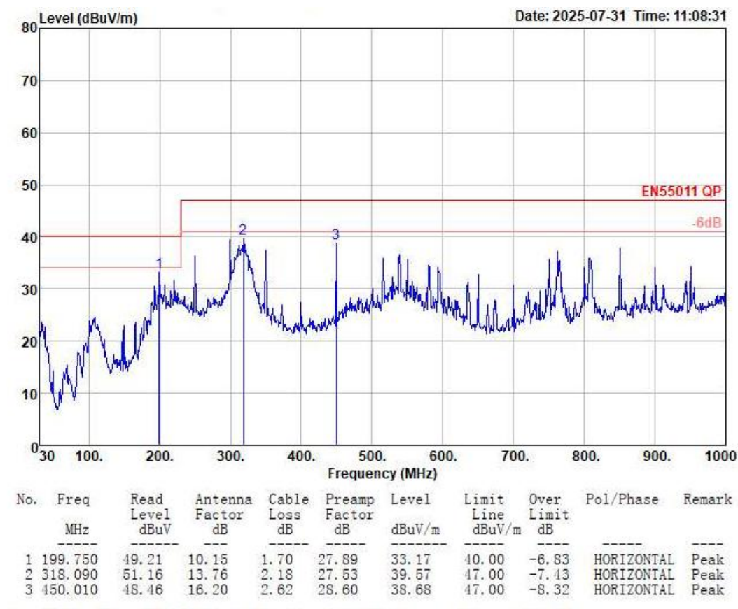
图 6-6 辐射测试水平方向
