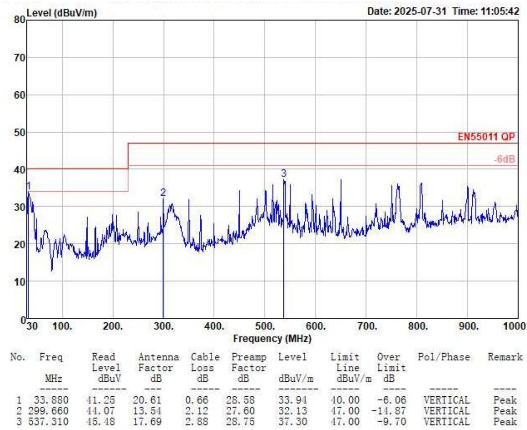
图 6-7 辐射测试垂直方向
