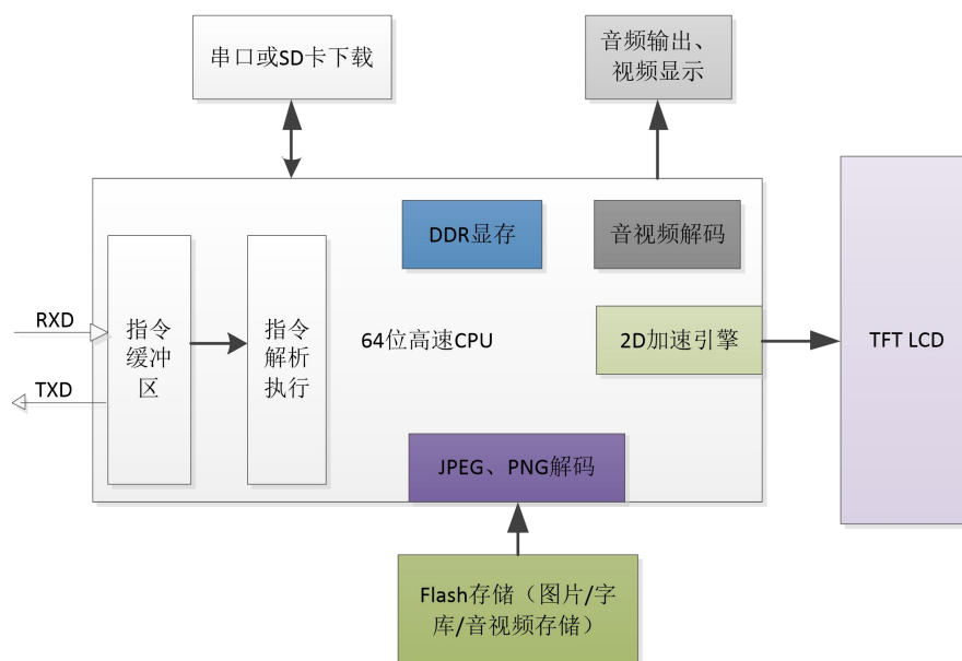
图 3-1 DH 系列串口屏内部结构图
