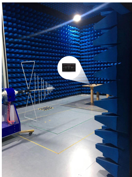
图 6-5 辐射测试图
